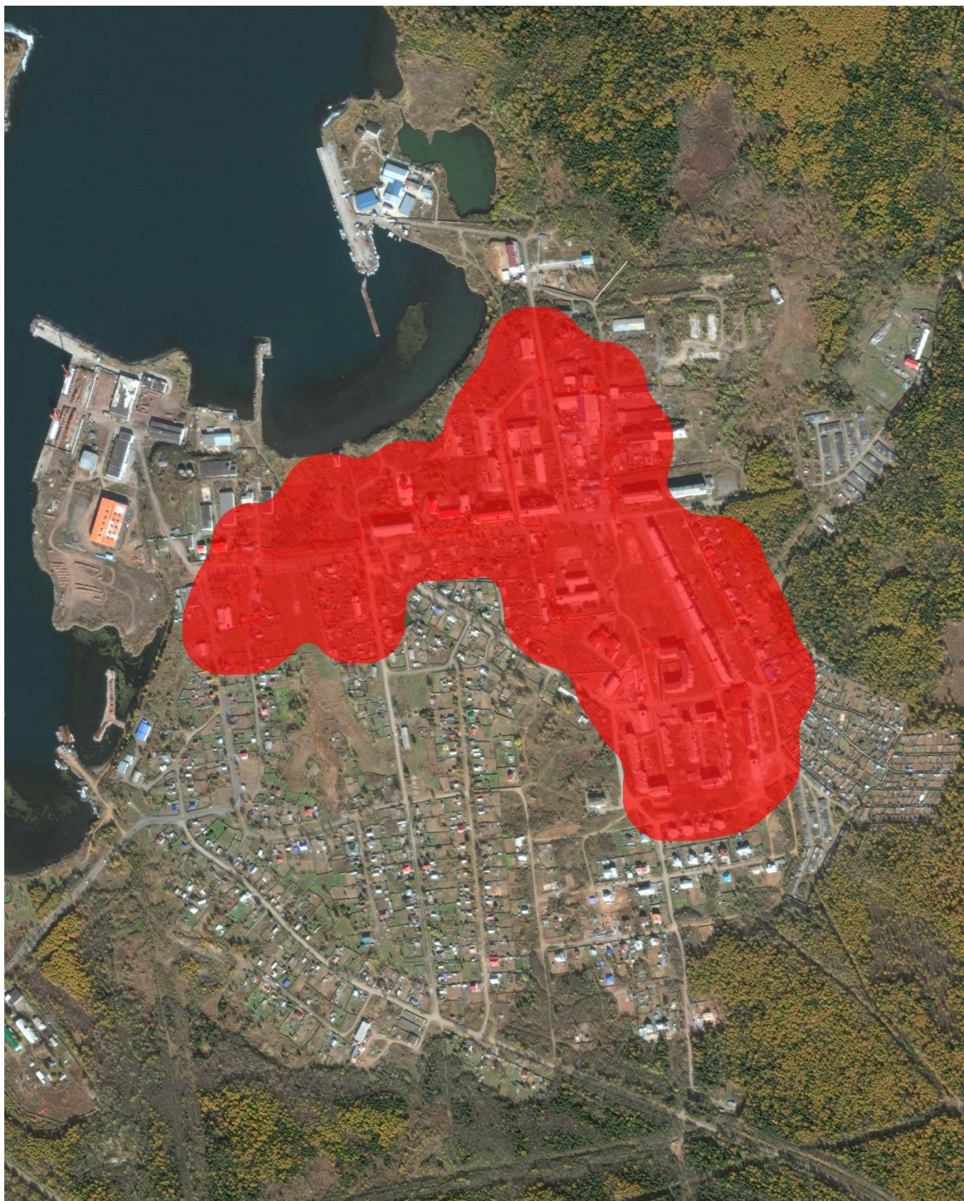
Рис. 2.1 – Зона действия системы теплоснабжения пгт. Лососина
