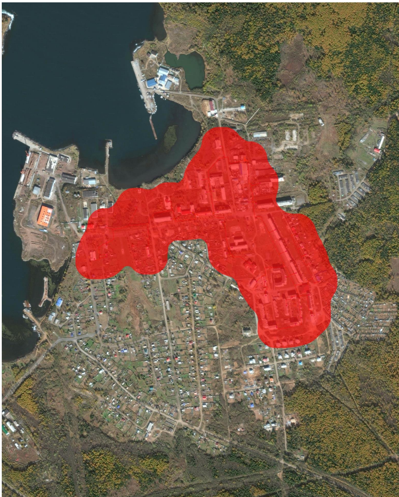
Рис. 1.1 - Зоны действия систем теплоснабжения муниципального образования «Рабочий поселок Лососина»
