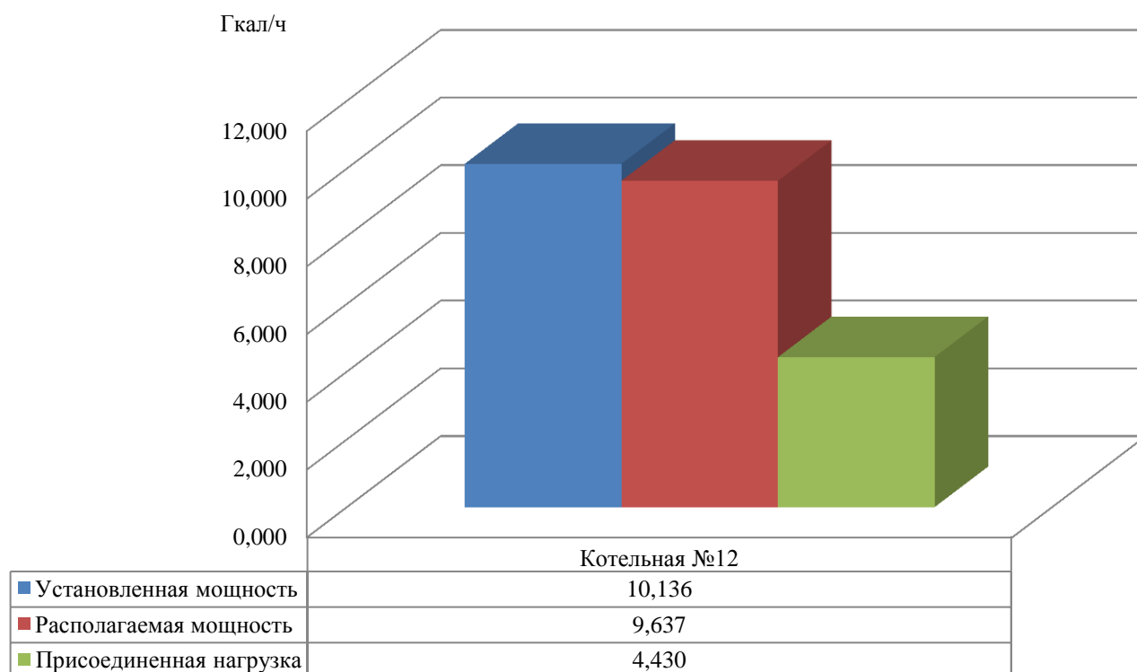
Рис. 1.2 – Распределение мощностей источников тепловой энергии
